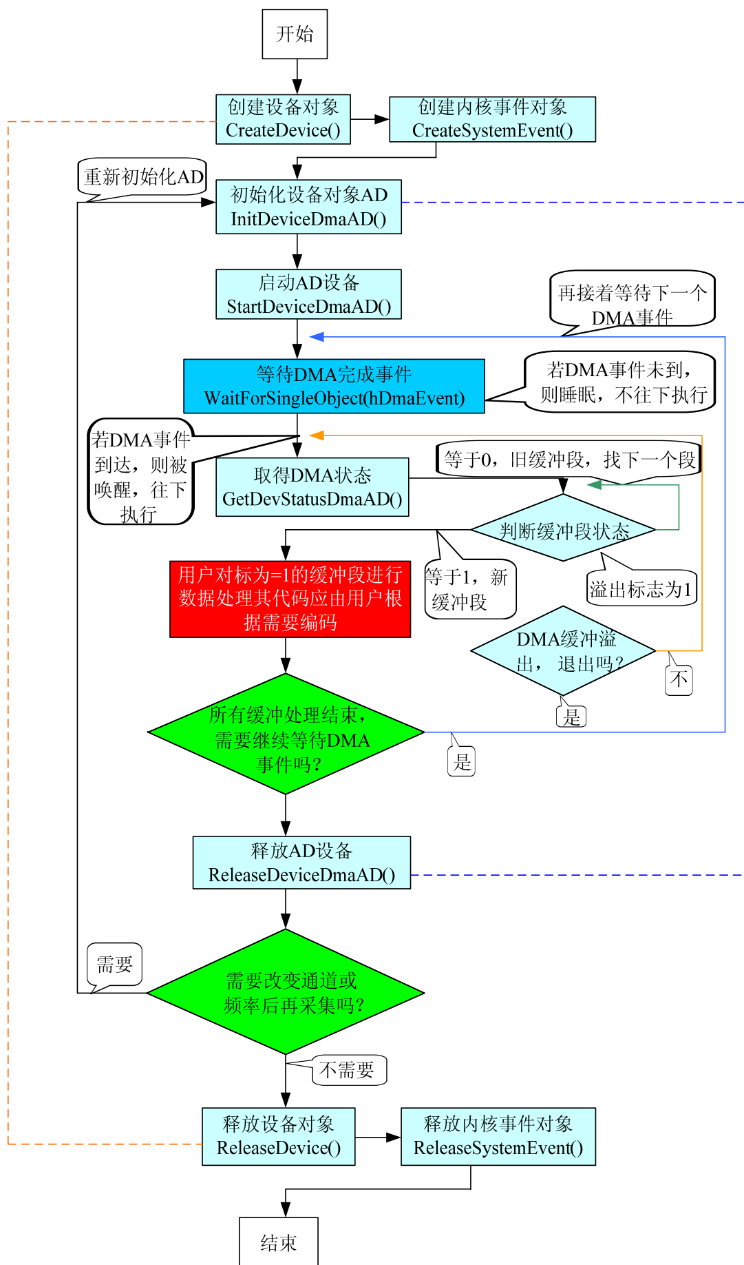
图 2.1.2 DMA 方式 AD 采集实现过程
