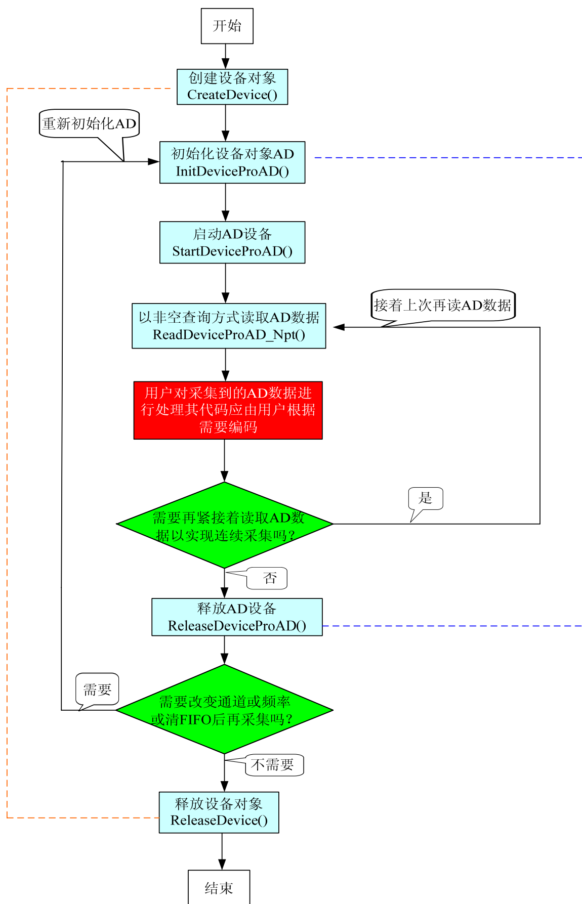
图 2.1.1 非空方式 AD 采集实现过程
