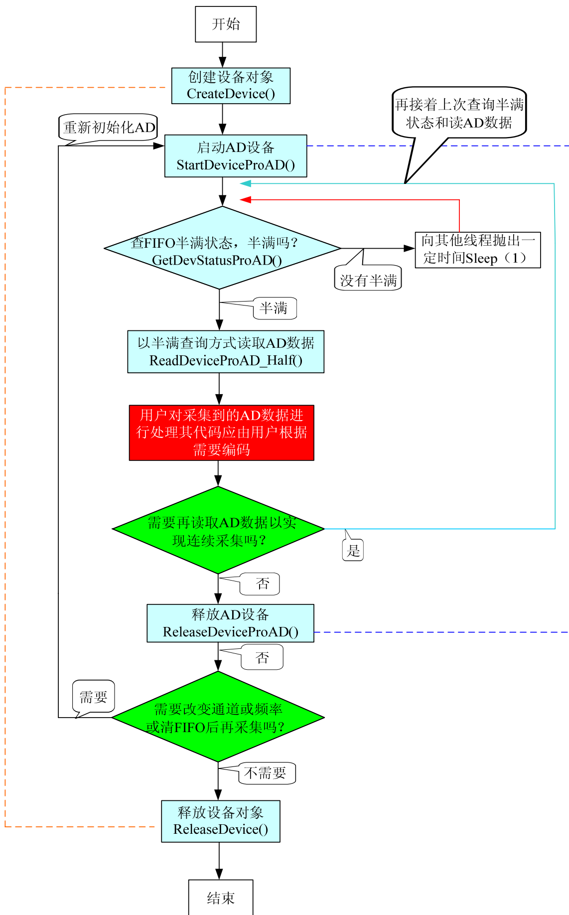
图 2.1.2 半满方式 AD 采集实现过程
