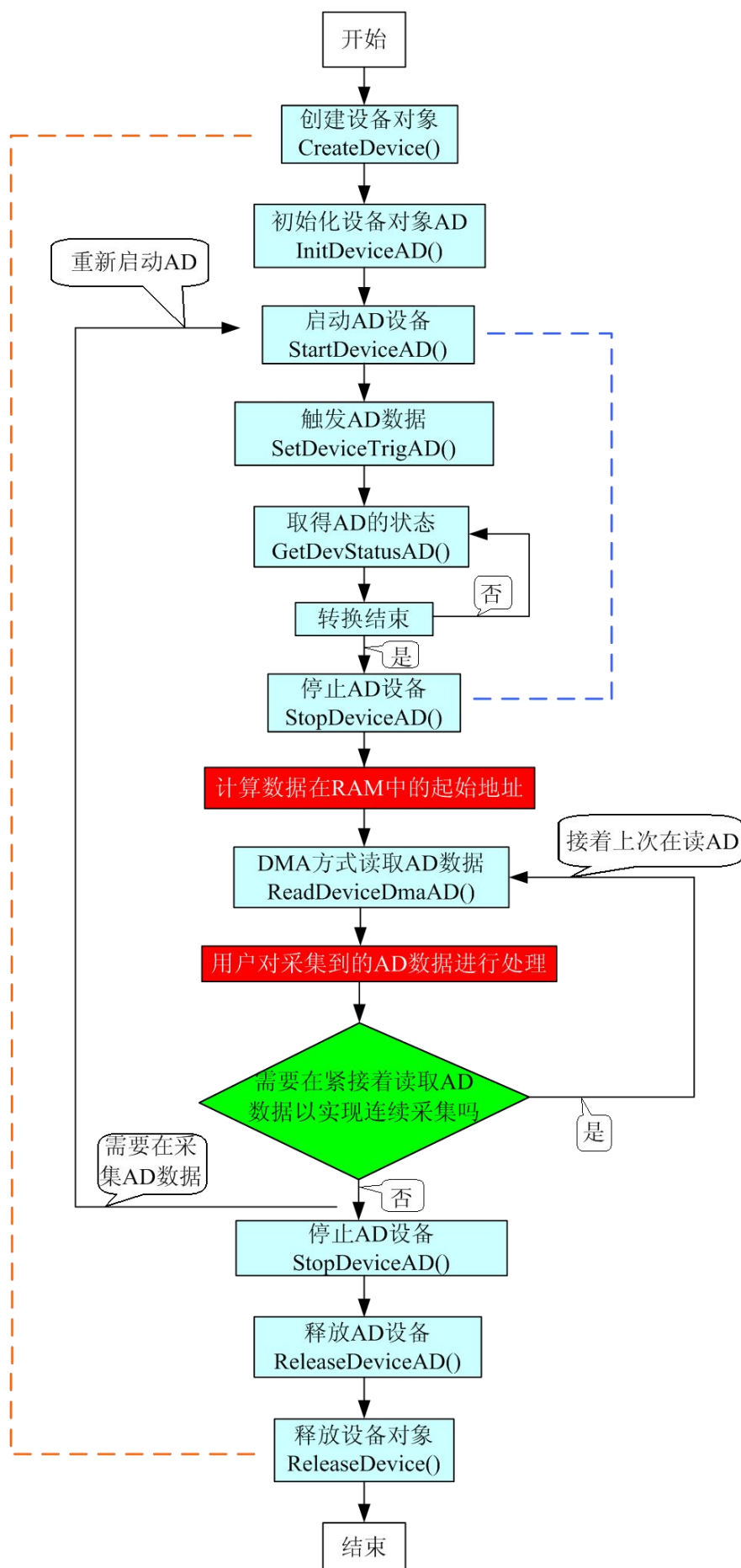
图 2.1.3 DMA 方式 AD 采集过程
