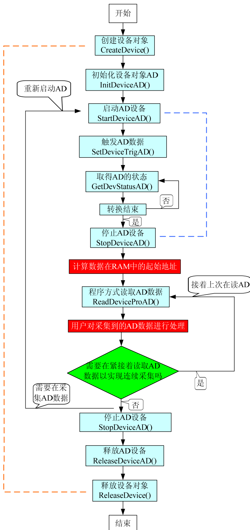
图 2.1.1 程序方式 AD 采集实现过程
